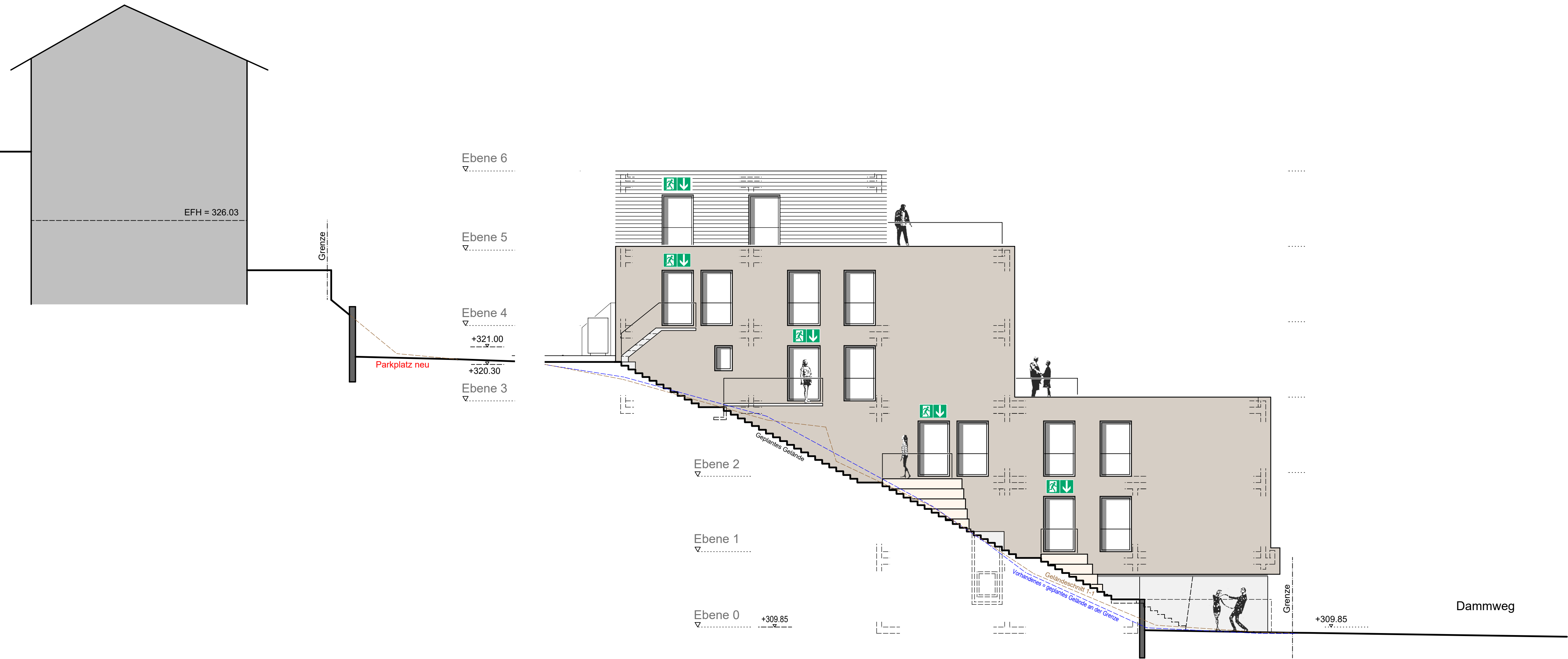
Ansicht Nord-Ost Geländeschnitt 1-1
