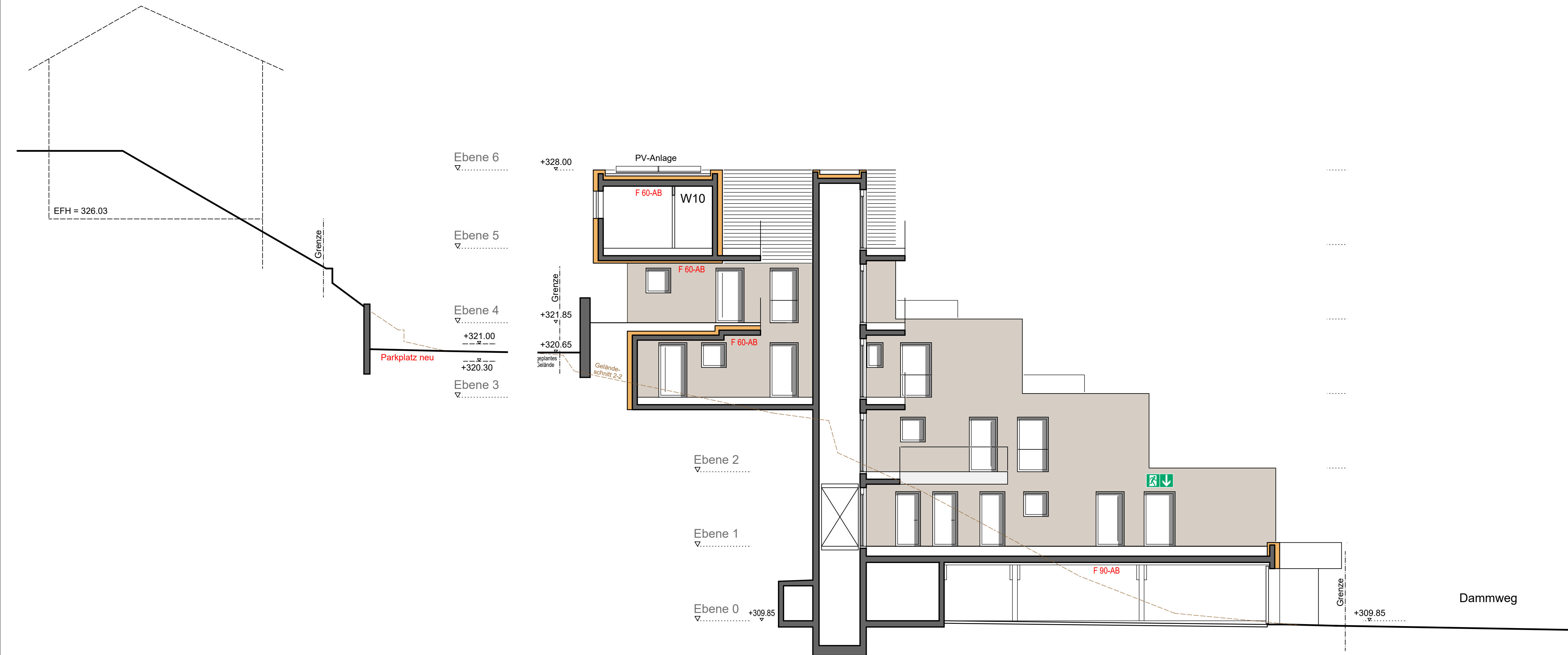
Schnitt C-C / Ansicht Nord-Ost Geländeschnitt 2-2
