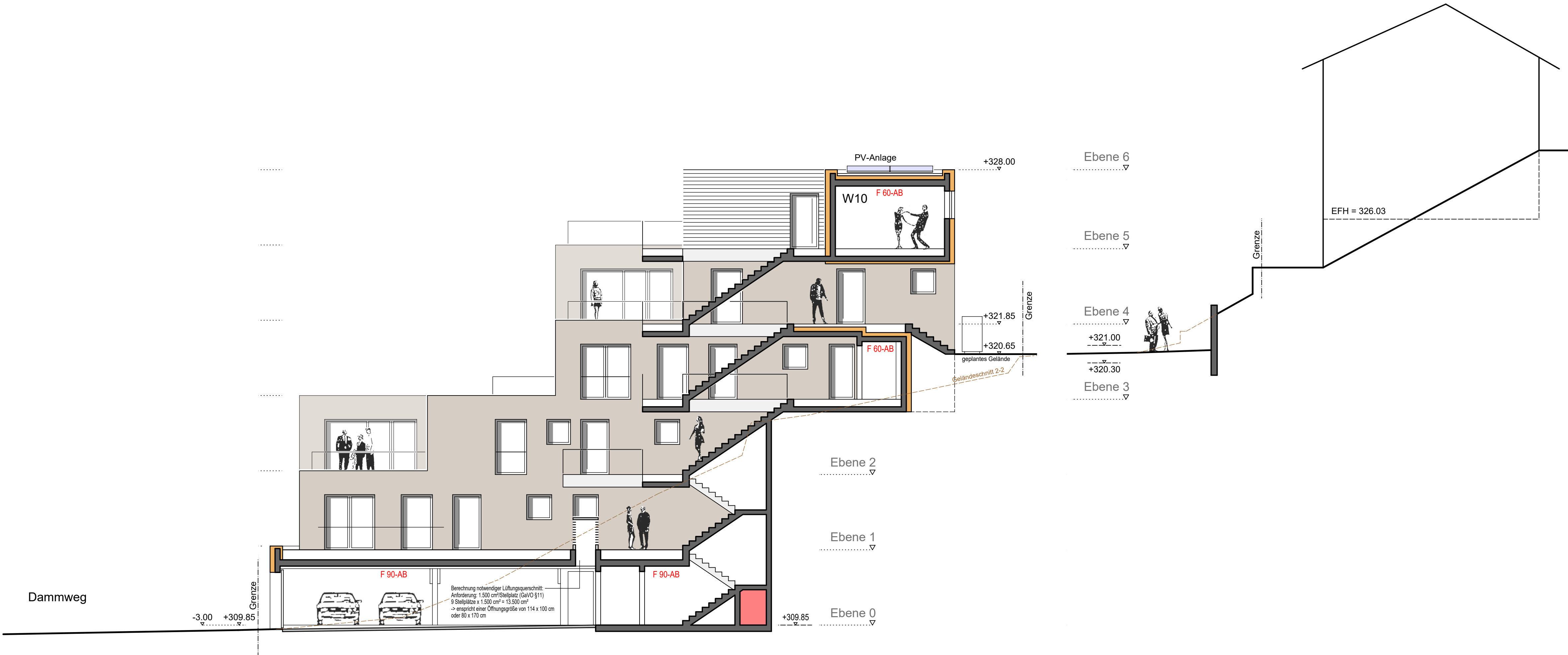
Schnitt B-B / Ansicht Süd-West Geländeschnitt 2-2
